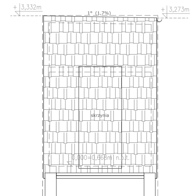
ELEWACJA PRZEDNIA (OD STRONY SAMOCHODU)
