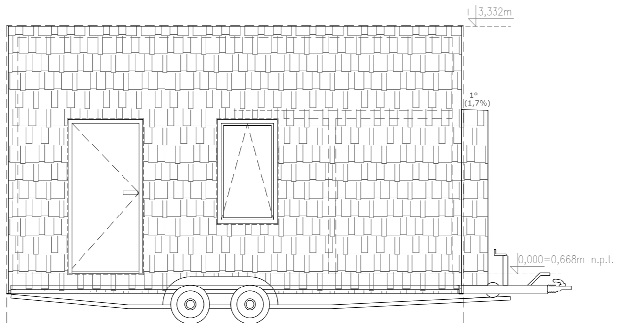
ELEWACJA BOCZNA (WEJŚCIOWA)
