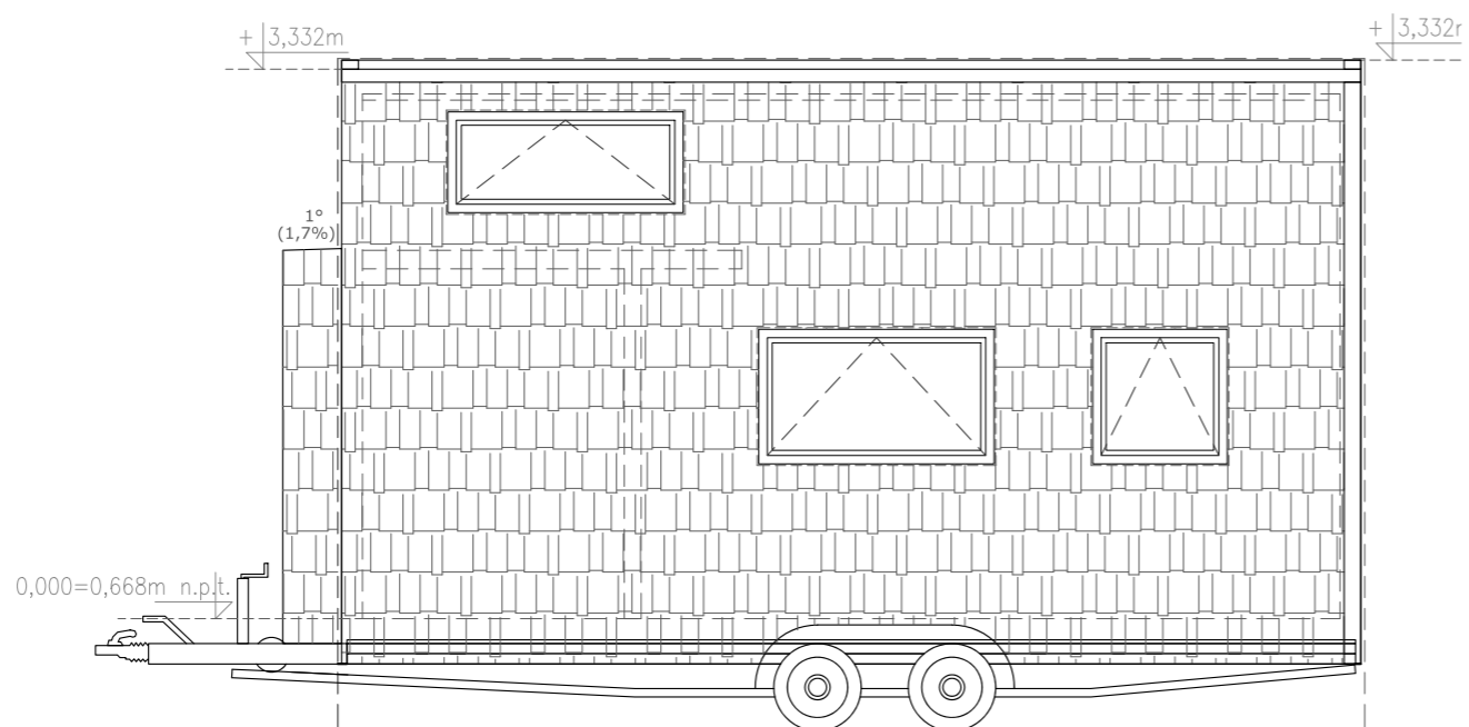
ELEWACJA BOCZNA
