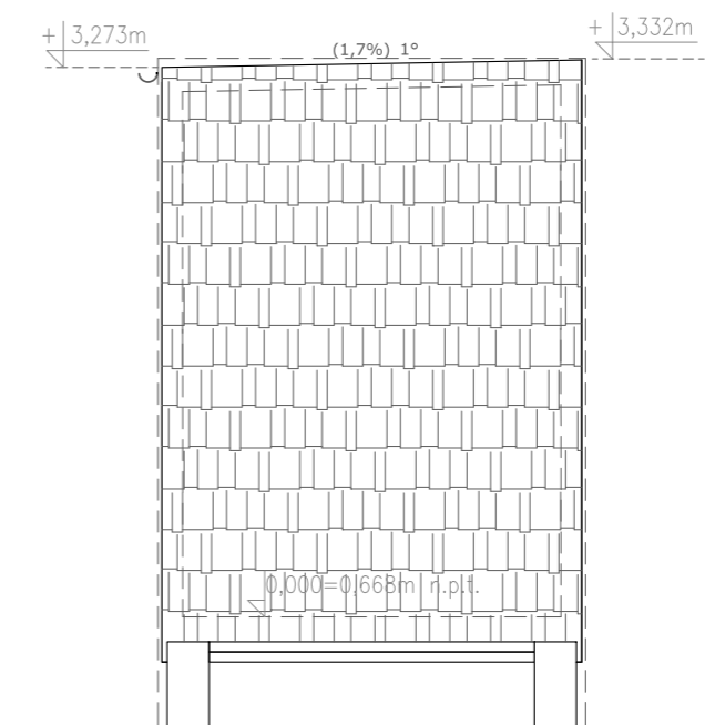
ELEWACJA TYLNA
